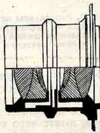
Рис. 9. Анастигмат
