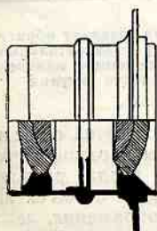
Рис. 8. Апланат
