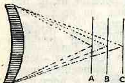
Рис. 1. Явление цветной aberrации в простой линзе (А — фокус синих лучей, В — фокус желтых лучей, С — фокус красных лучей)
