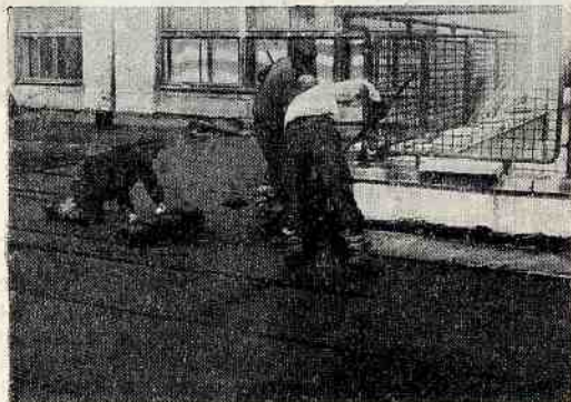
РАБОТЫ ПО ХОЛЬЦ-ЦЕМЕНТУ
