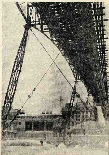
Эстокада Шатурской электростанции — А. Алексеев (Ленинград).
